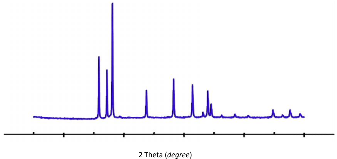
Gambar 4 ZnO doped Cu 2+ 3%.
