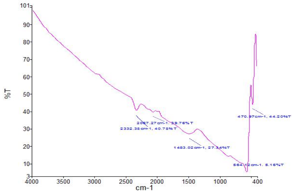
Gambar 1. Spektra FTIR ZnO doped Cu 3%.
